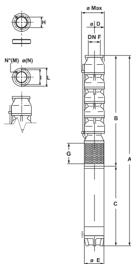
Overall dimensions and weights / Dimensions d'encombrement et poids Dimensioni di ingombro e pesi
