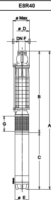
Overall dimensions and weights Dimensions d'encombrement et poids Dimensioni di ingombro e pesi
